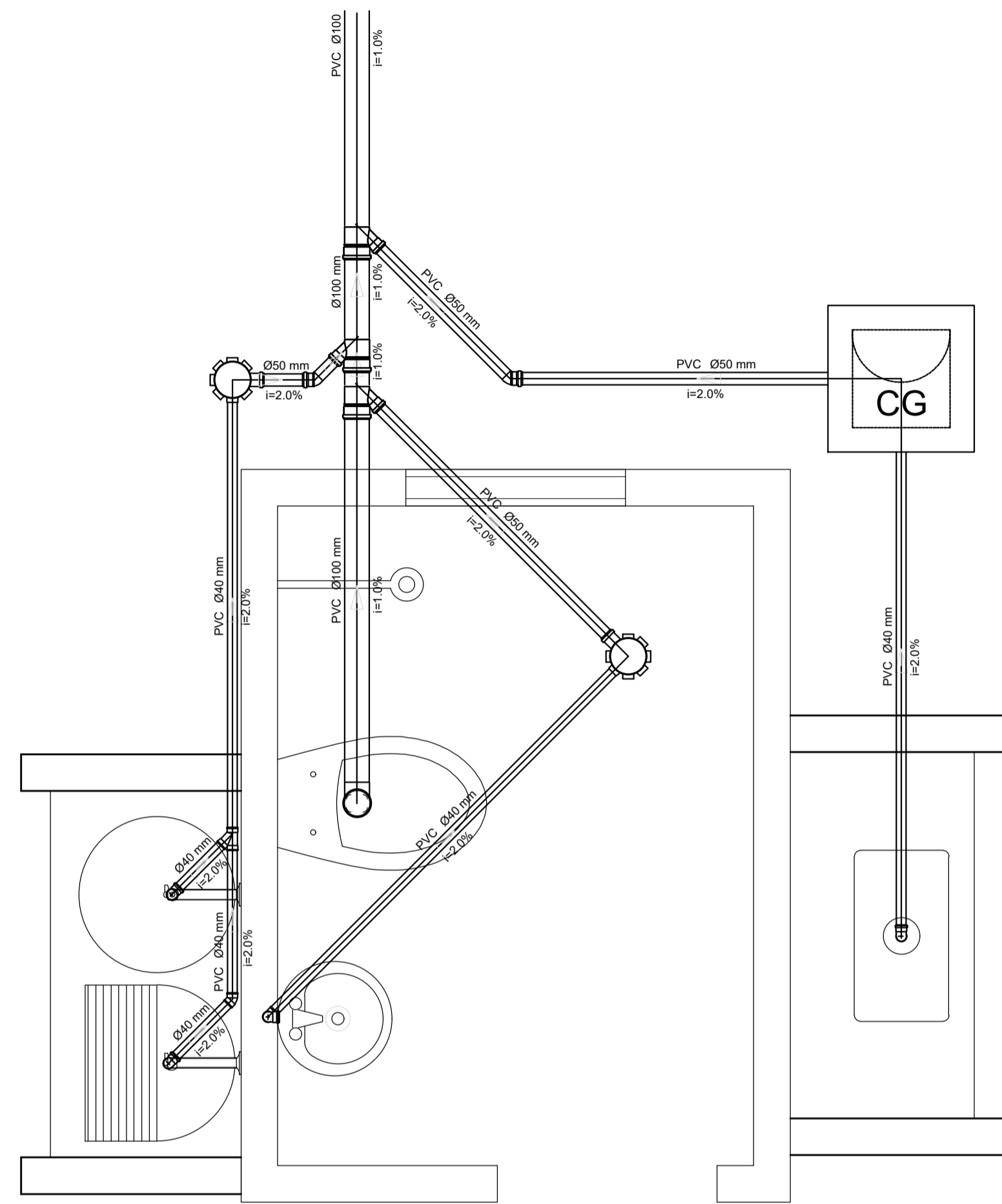
1 PLANTA BAIXA ESCALA 1:20
