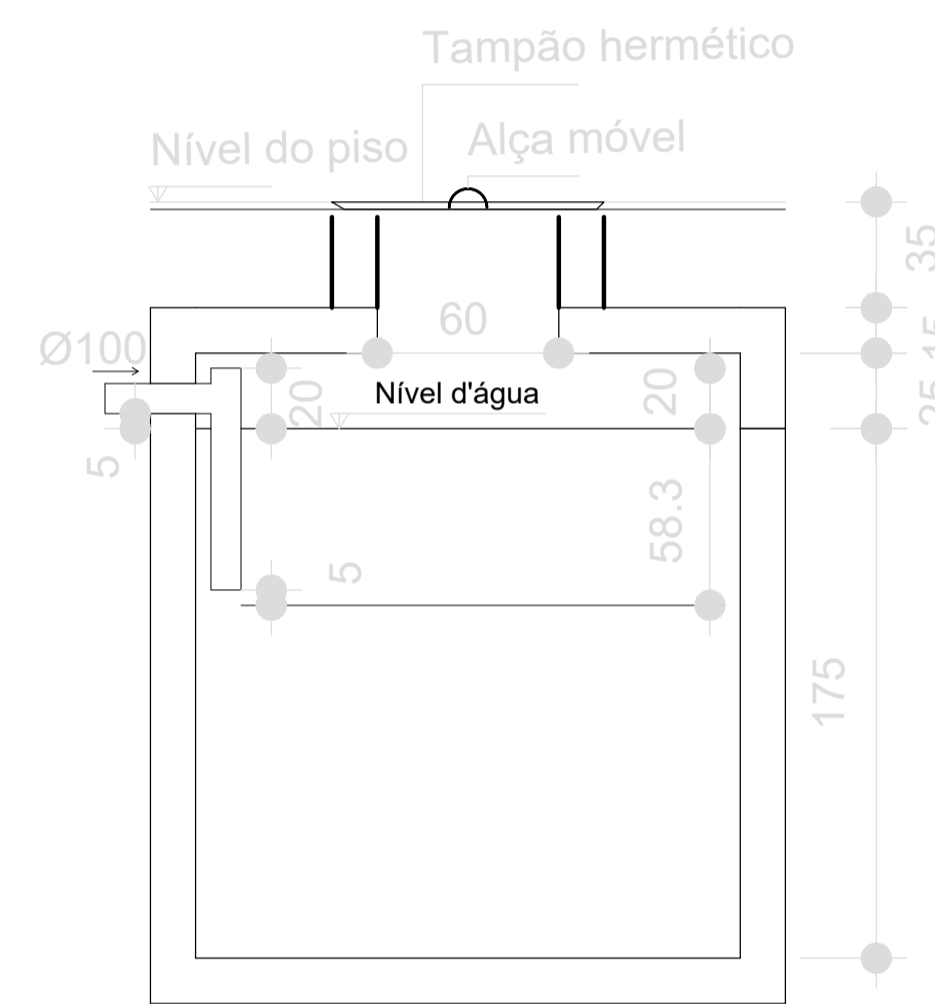
5 TANQUE SÉPTICO CORTE ESCALA 1:25
