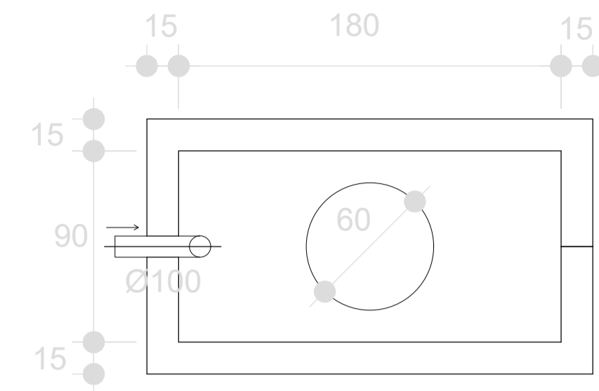
4 TANQUE SÉPTICO PLANTA BAIXA ESCALA 1:25
