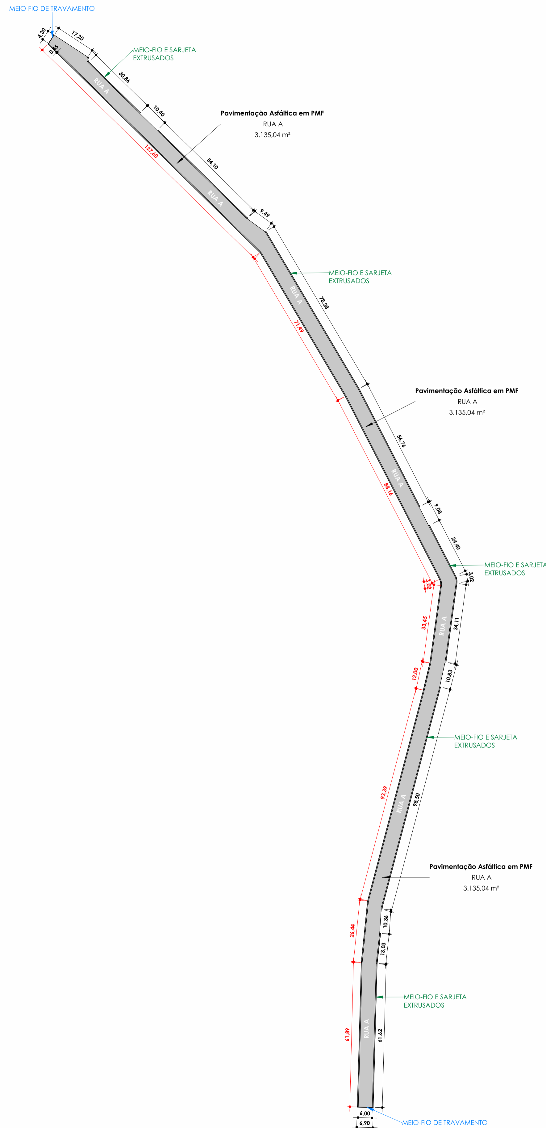
PLANTA DE COTAS - RUA A ESC: 1 : 1000
