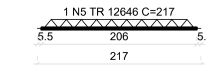
VT7a (4 unidades) (L7) ESC 1:50
