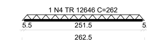
VT10a (9 unidades) (L10) ESC 1:50
