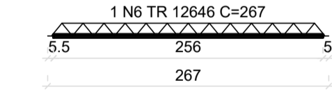
VT14a (7 unidades) (L14) ESC 1:50
