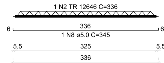
VT4b (12 unidades) (L4) ESC 1:50
