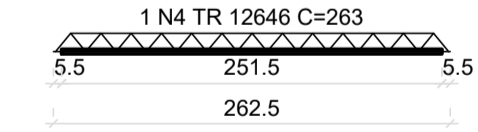
VT11a (9 unidades) (L11) ESC 1:50
