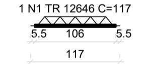
VT12a (3 unidades) (L12) ESC 1:50
