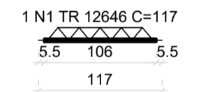
VT4a (2 unidades) (L4) ESC 1:50
