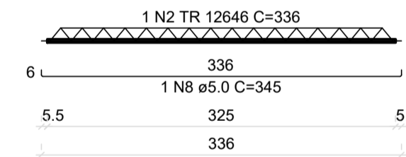
VT1b (12 unidades) (L1) ESC 1:50
