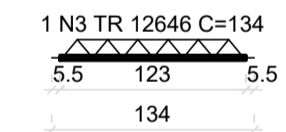
VT3a (5 unidades) (L3) ESC 1:50
