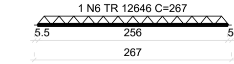
VT13a (7 unidades) (L13) ESC 1:50
