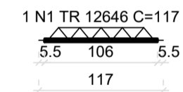
VT1a (2 unidades) (L1) ESC 1:50
