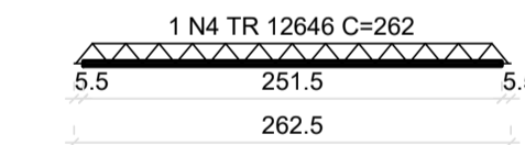
VT5a (6 unidades) (L5) ESC 1:50
