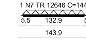
VT15a (5 unidades) (L15) ESC 1:50
