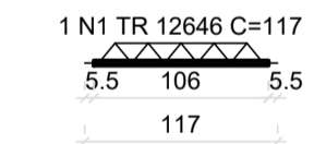
VT9a (3 unidades) (L9) ESC 1:50
