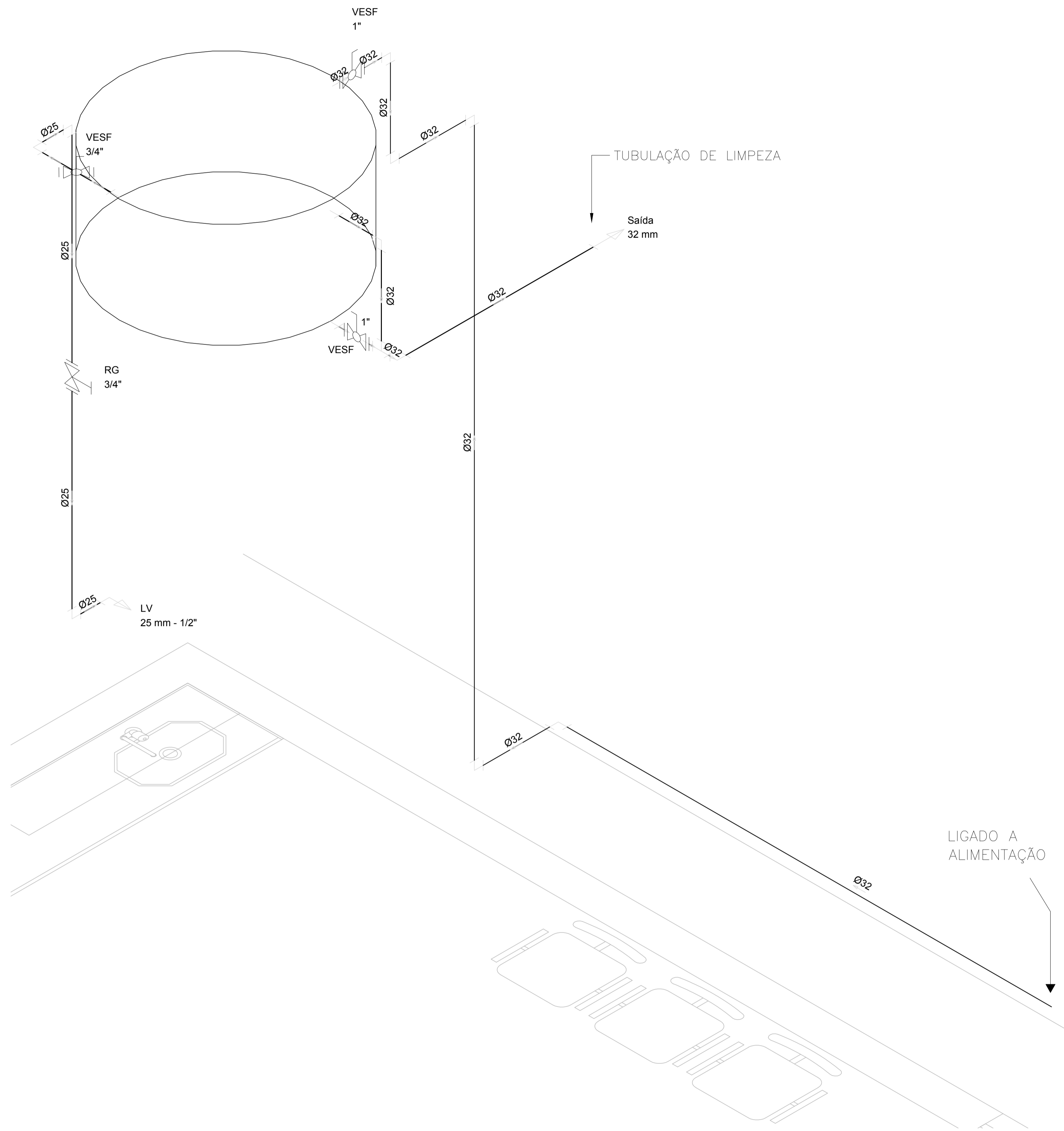
1 DETALHE ISOMÉTRICO ESCALA 1:50
