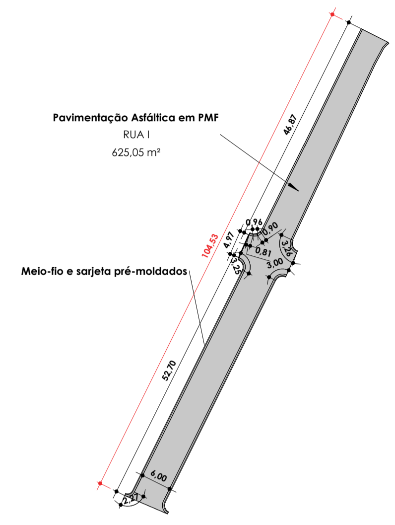
PLANTA DE COTAS - RUA I ESC:1 : 750
