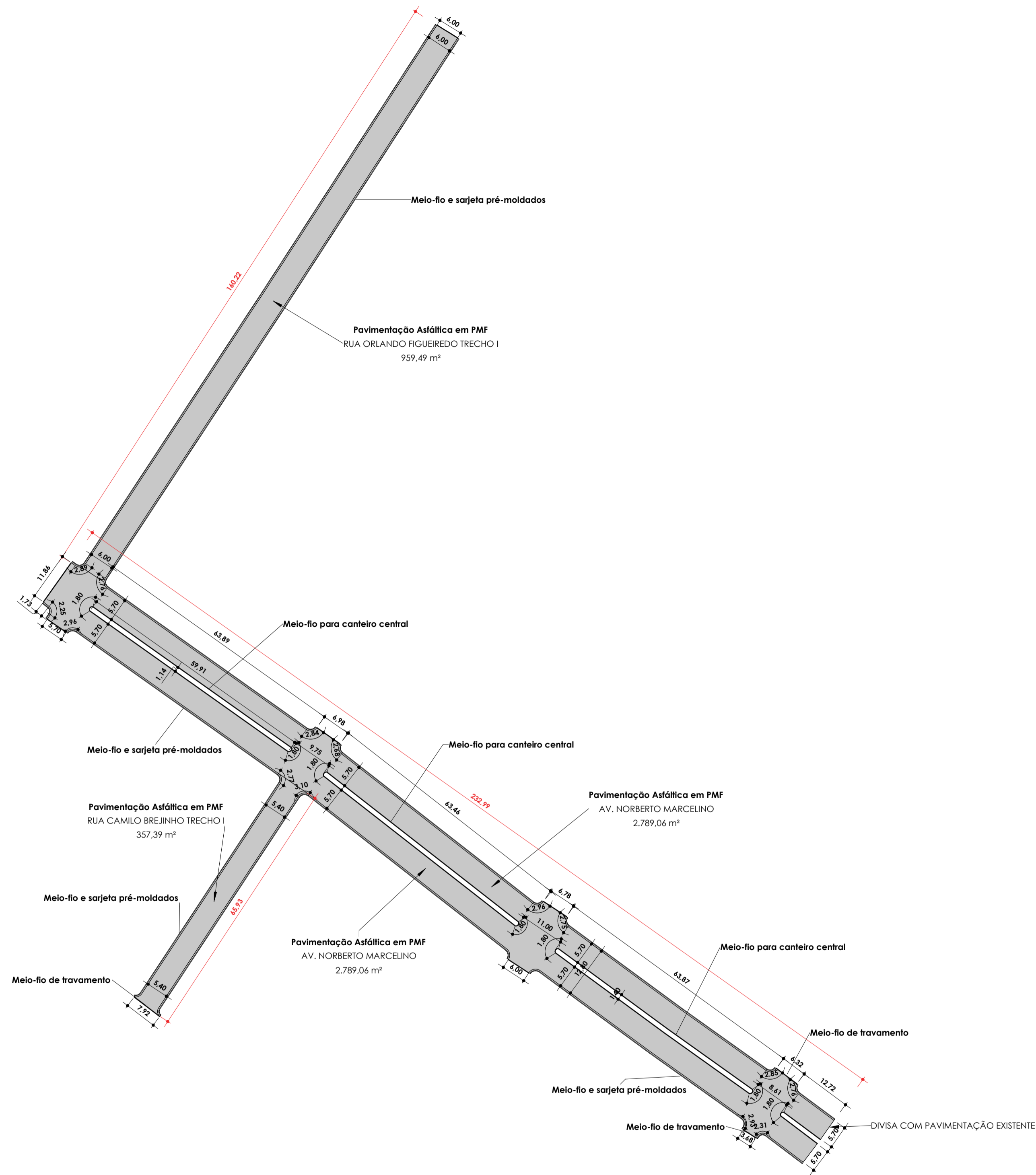
PLANTA DE COTAS - RUA ORLANDO FIGUEIREDO TRECHO I, AV. NORBERTO MARCELINO, RUA CAMILO BREJINHO TRECHO I ESC:1 : 750
