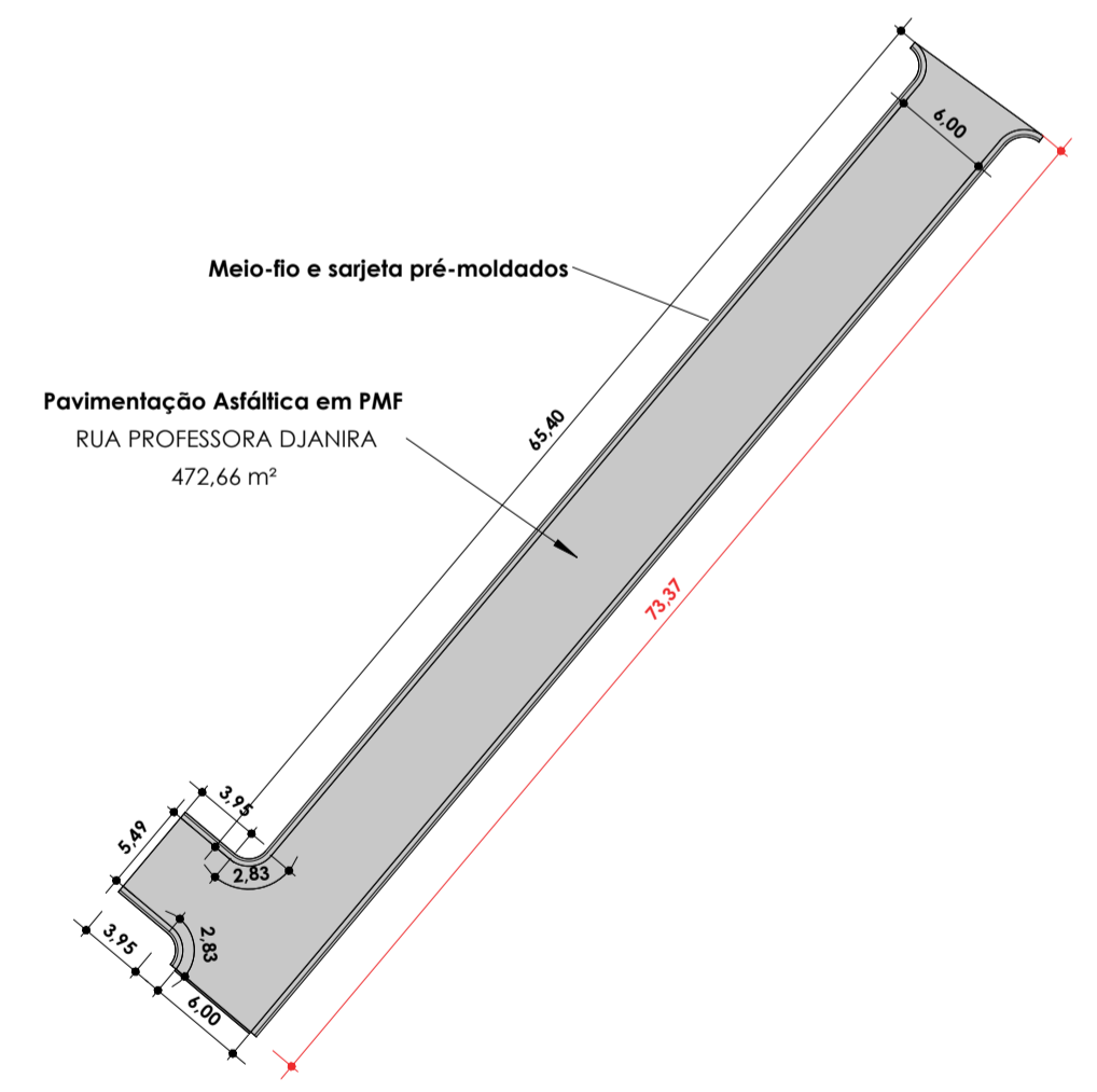
PLANTA DE COTAS - RUA PROFESSORA DJANIRA ESC: 1 : 500
