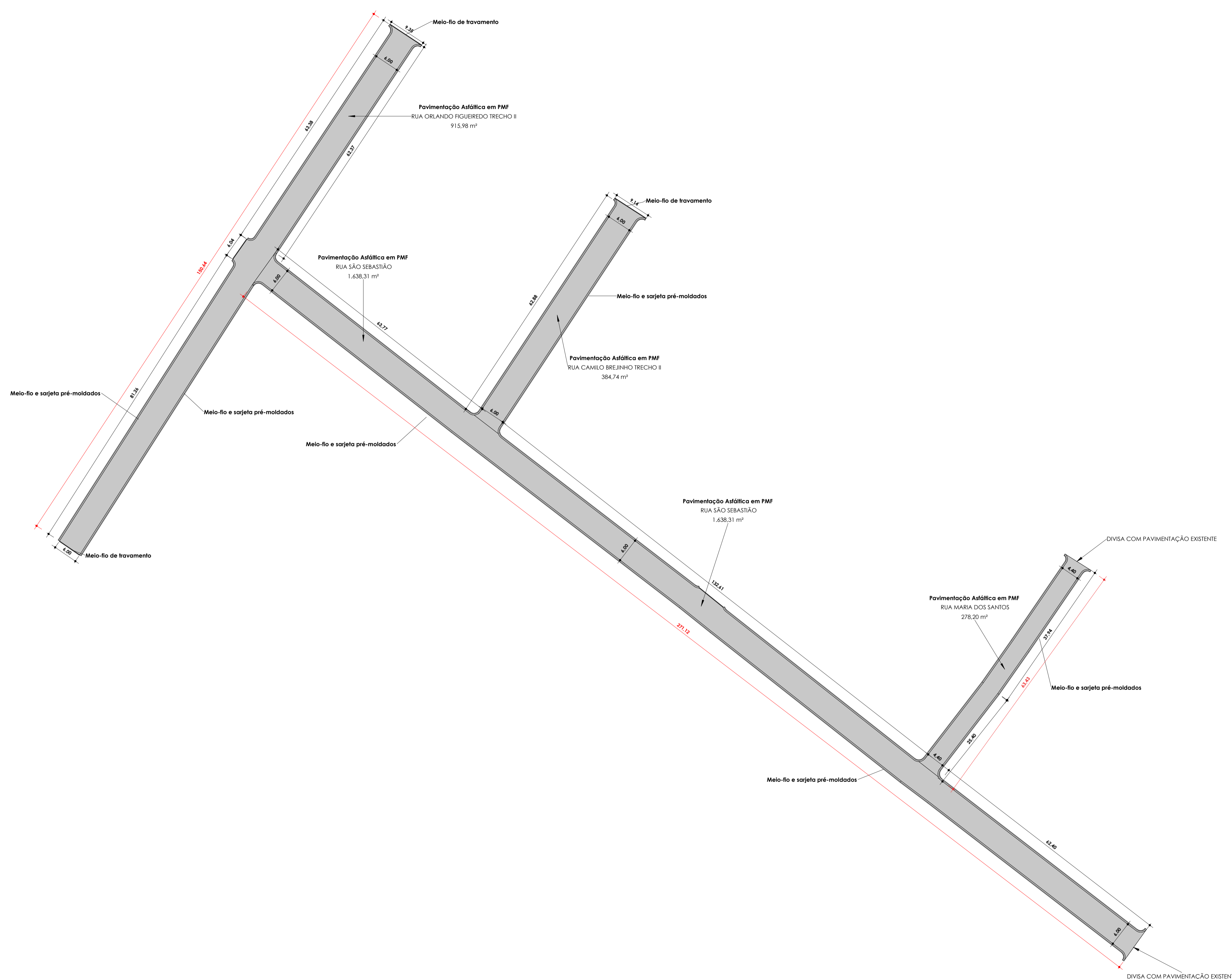
PLANTA DE COTAS - RUA ORLANDO FIGUEIREDO TRECHO II, RUA SÃO SEBASTIÃO, RUA CAMILO BREJINHO TRECHO II E RUA MARIA DOS SANTOS ESC: 1 : 500
